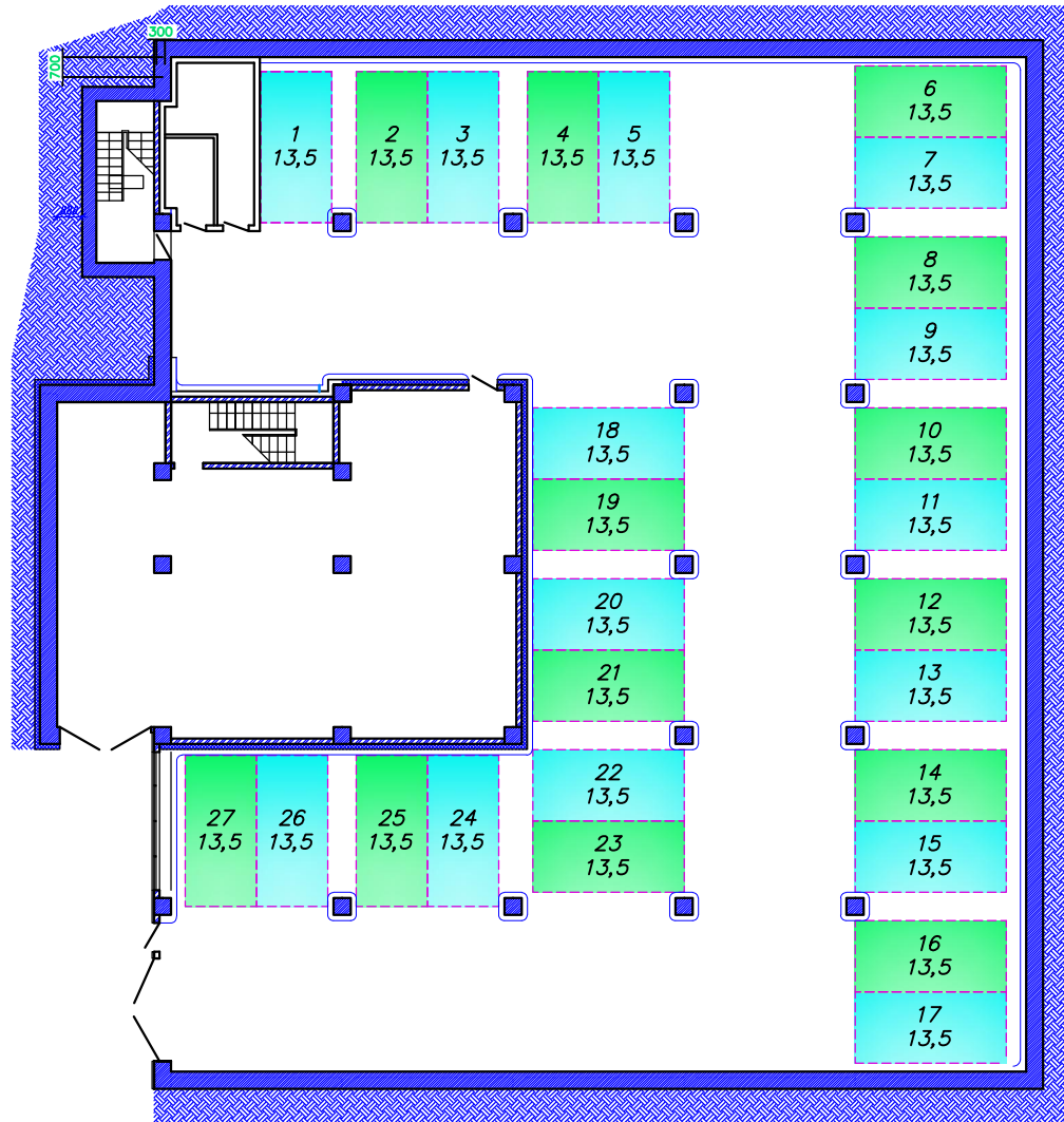
План отм. 0.000
